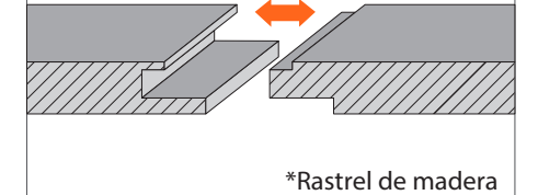
PERFIL MACHIEMBRADO MALE-FEMALE JOINT
