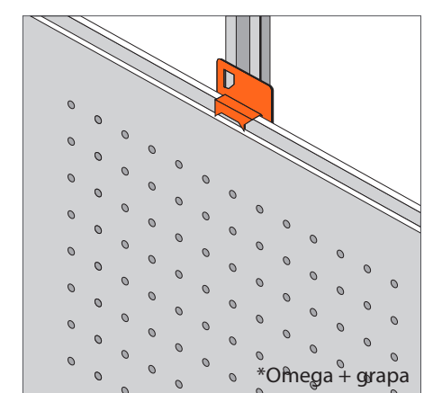
PERFIL MACHIEMBRADO MALE-FEMALE JOINT
