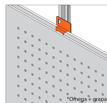
PERFIL MACHIHembrado MALE-FEMALE JOINT ■ Omega + grapa ■ Rastrel de madera
