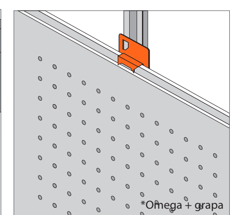
PERFIL MACHIEMBRADO MALE-FEMALE JOINT *Omega + grapa *Rastrel de madera
