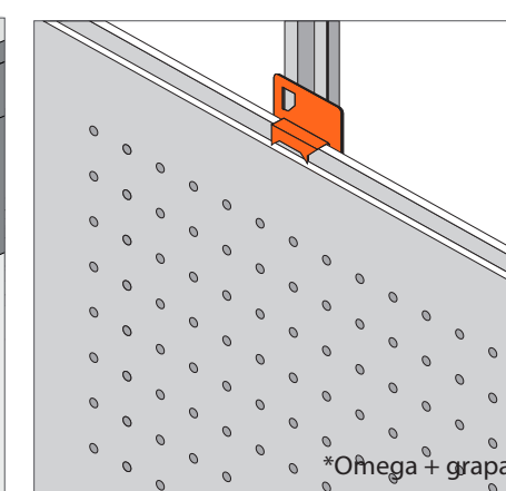
PERFIL MACHIEMBRADO MALE-FEMALE JOINT
