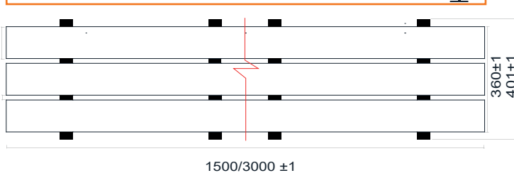
Vista inferior | Bottom view
