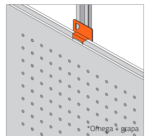
PERFIL MACHIHERRADO MALE-FEMALE JOINT ■ Omega + grapa ■ Rastrel de madera *Rastrel de madera
